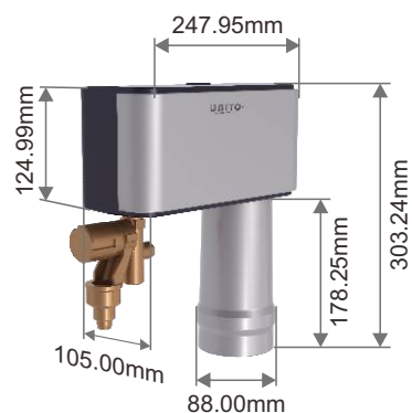
UNITO koeler
